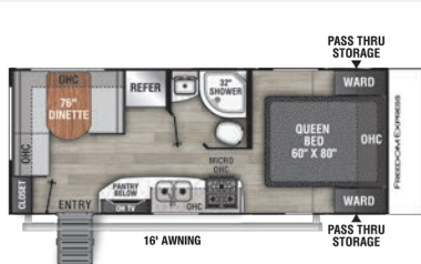
20 SE / Exterior Length 24' 6"
