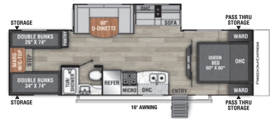
29 SE / Exterior Length 33' 4"
