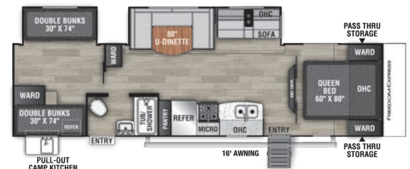
31 SE / Exterior Length 35' 6"
