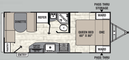
204 RD / Exterior Length 24' 7"
