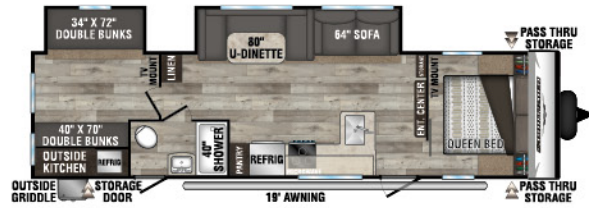
312BHKSE UVW - 6,900 | Exterior Length - 35'9\"/>
