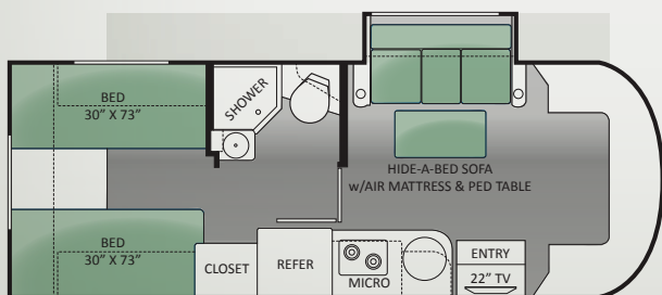
CITATION SPRINTER 24ST
