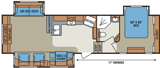
35RE • UVW TBD • Dry Hitch Wt. TBD • NCC TBD • Length 36'9"
