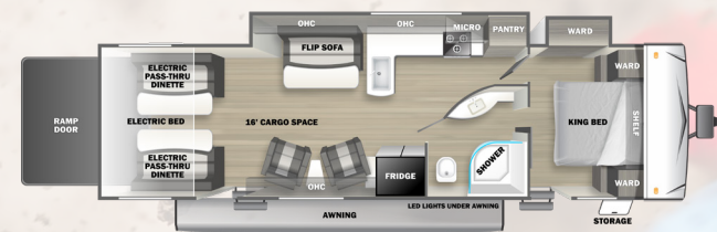
304GSLR (16' CARGO)
