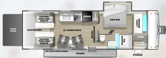
265GSLR (16' CARGO)
