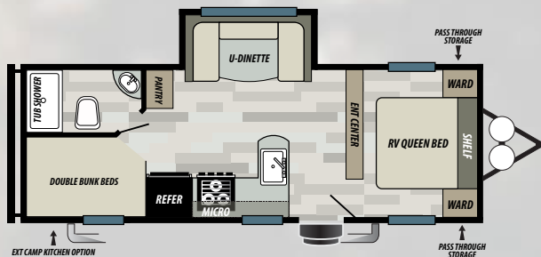
241BHXL
