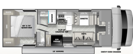
2951SLE (Available on Ford E450)
