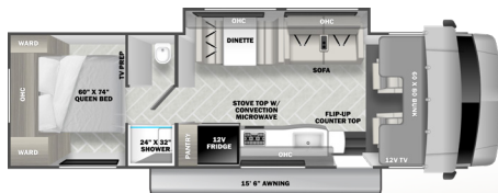
2851SLE (Available on Ford E450)
