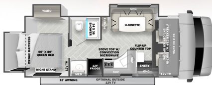
2501TS (Available on Ford E450)
