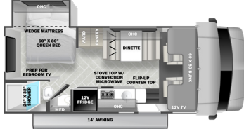
2251SLE (Available on Ford E350/Chevy 3500)
