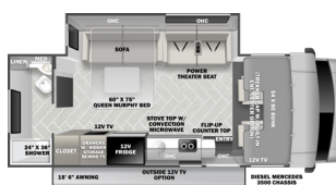
2401T (Available on Sprinter 3500)
