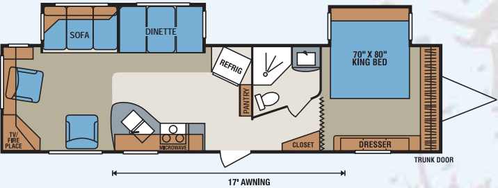
D330RE • UVW 8136 • Dry Hitch Wt. 1160 • NCC 2064 • Length 37'6"
