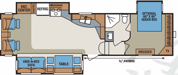
D3255PX3 • UVW 9644 • Dry Hitch Wt. 1967 • NCC 4156 • Length 34'9"
