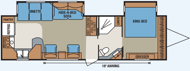
D321RK • UVW 8259 • Dry Hitch Wt. 1046 • NCC 1741 • Length 36'
