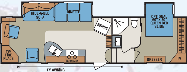
D305SB • UVW 8628 • Dry Hitch Wt. 1975 • NCC 2172 • Length 32'9"
