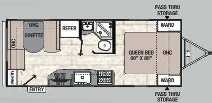
204 RD / Exterior Length 24' 7"
