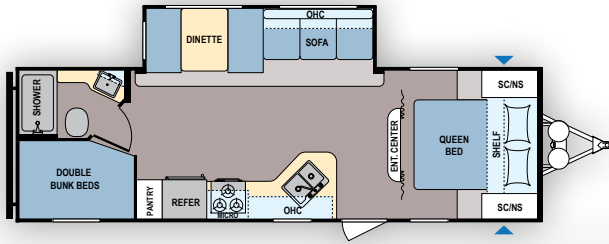
Lantern | 262BH
