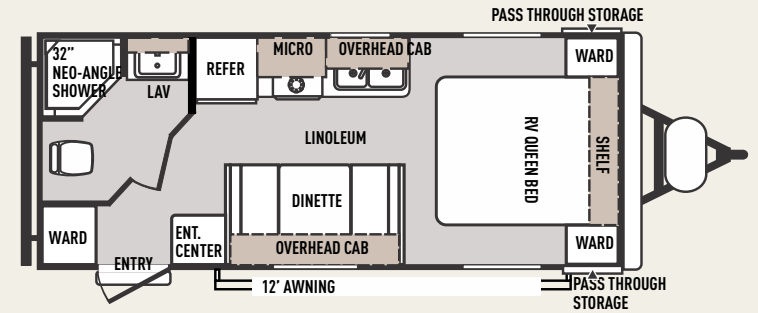
221RBXL
