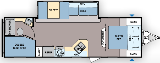
Lantern | 262BH
