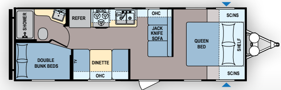
Lantern | 274BH
