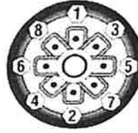
8-Lug Nuts
